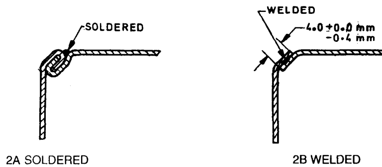
FIG. 2 SIDE SEAM
